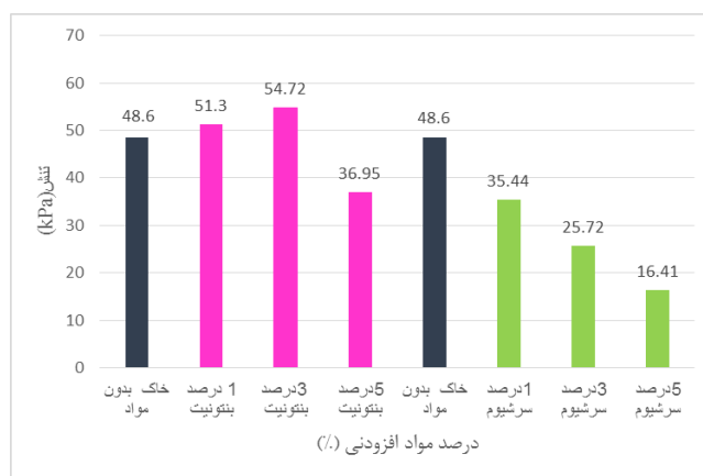
شکل ۶. تأثیر درصد‌های وزنی مختلف بنتونیت و سريشم بر روی مقاومت فشاری خاک رسی
