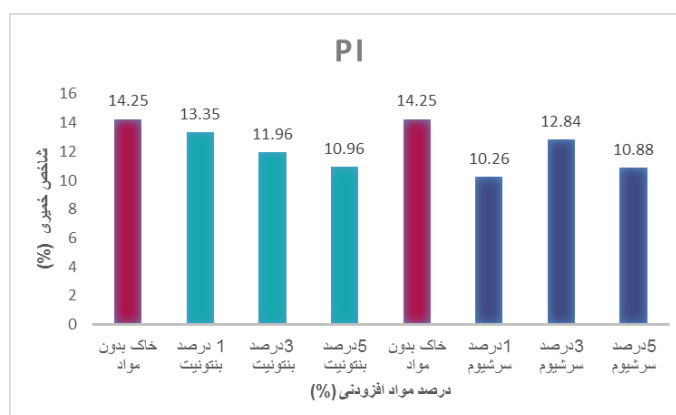
شکل ۴- تأثیر درصدهای وزنی مختلف بنتونیت و سریشیم بر روی شاخص خمیری خاک
