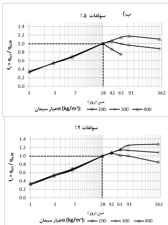
شکل ۱۰. تغییرات مقدار پارامتر f_c در سنین مختلف به ازای عیارهای مختلف سیمان (200, 300, 400 \text{ kg/m}^3) و (200, 300, 400 \text{ kg/m}^3) (در سولفات الف) ۵٪ و ب) ۲٪.
