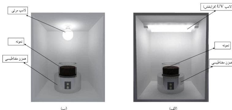
شکل ۱. شماتیکی از سیستم تابش امواج الکترومغناطیس روی نمونه‌های گل اشباع درون محفظه‌ای با فضای داخلی کاملاً تاریک (الف) نمونه روی هم‌زن مغناطیسی تحت تابش امواج فرابنفش در محدوده ۲۵۶-۳۶۰ nm، (ب) نمونه روی هم‌زن مغناطیسی تحت تابش امواج مرئی در محدوده ۴۰۰-۷۰۰ nm
