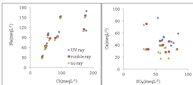
شکل ۶. نمودارهای ترکیبی کلر در برابر سدیم و سولفات در برابر کلسیم براساس نمونه‌های تحت اثر بخشی امواج فرابنفش (UV)، امواج مرئی (visible) و روش استاندارد (no ray)
