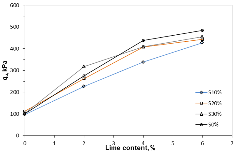
شکل ۸. اثر مقادیر مختلف آهک بر مقاومت فشاری نمونه‌های بهسازی شده با مقادیر مختلف سرباره
