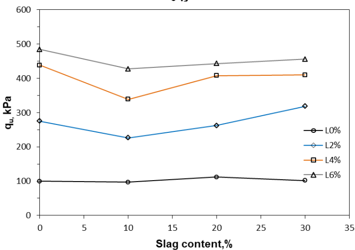
شکل ۹. اثر مقادیر مختلف سرباره بر مقاومت فشاری نمونه‌های بهسازی شده با مقادیر مختلف آهک
