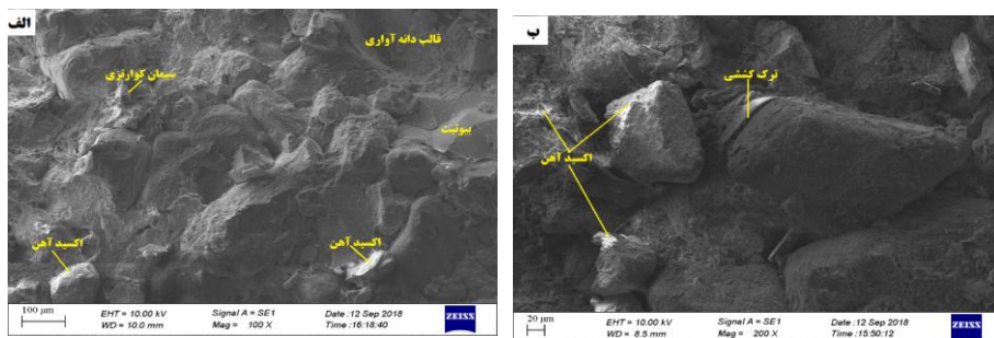
شکل ۸. تصاویر SEM از سطح شکست نمونه GD1، الف-ج) و نمونه GD2، د)
