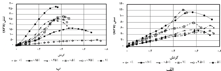
شکل ۷. تأثیر مقادیر مختلف نانوذرات بر مقاومت فشاری محصورنشده خاک بهسازی شده با (الف) نانورس (ب) نانوسیلیکا
