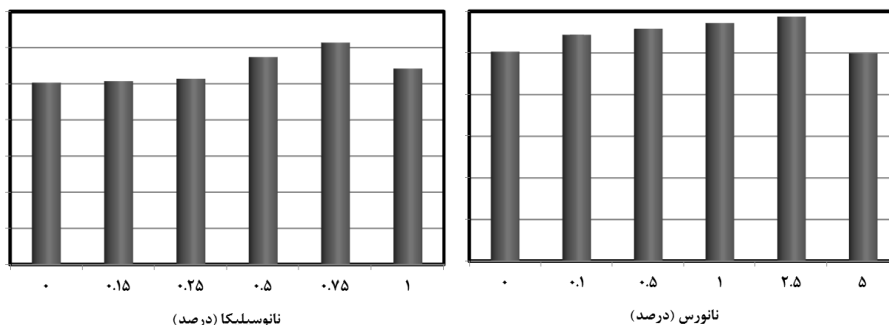
شکل ۵. مقایسه تغییرات زاویه اصطکاک داخلی در خاک‌های به‌سازی شده با نانوس و نانوسیلیکا
