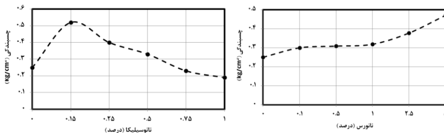
شکل ۶. مقایسه تغییرات چسبندگی در خاک‌های به‌سازی شده با نانوس و نانوسیلیکا
