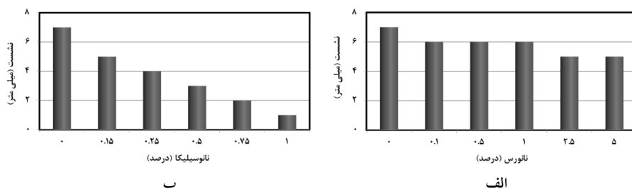
شکل ۸. تأثیر مقادیر مختلف نانوذرات بر تغییرات نشست پذیری خاک بهسازی شده با (الف) نانورس (ب) نانوسیلیکا
