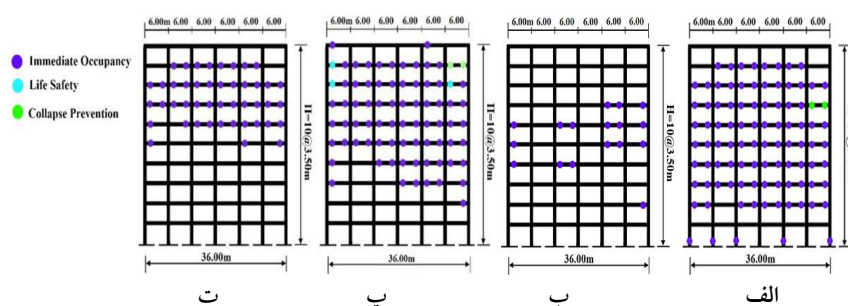
شکل ۱۵. محل و آرایش تشکیل مفاصل پلاستیک در مدل ۱۰ طبقه با توجه به حدود تعریف شده در Fema 356: الف) و ب) مدل تحت رکورد مقیاس شده طیس ۱۹۷۸ بر اساس استاندارد ۳-۲۸۰۰ و ۴-۲۸۰۰، پ) و ت) مدل تحت رکورد مقیاس شده نورتریج-رینالدی ۱۹۹۴ بر اساس استاندارد ۳-۲۸۰۰ و ۴-۲۸۰۰
