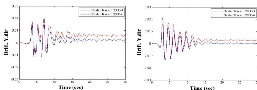
شکل ۱۷. تاریخچه زمانی دررفت طبقه بام مدل ۱۰ طبقه تحت اثر دو رکورد، الف) رکورد بام، ب) رکورد SCE
