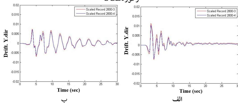
شکل ۱۸. تاریخچه زمانی دررفت طبقه بام مدل ۲۰ طبقه تحت اثر دو رکورد، الف) رکورد بام، ب) رکورد SCE
