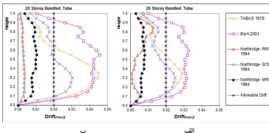
شکل ۱۴. پوش بیشینه جا به جایی نسبی طبقات مدل ۲۰ طبقه در نقطه D پلان، الف) نمایش گر پاسخ سازه تحت رکوردهای مقیاس شده بر اساس ویرایش سوم است، ب) نیز نمایش گر پاسخ سازه تحت رکوردهای مقیاس شده بر اساس ویرایش چهارم آیین نامه ۲۸۰۰ است
