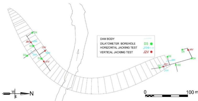
شکل ۳. موقعیت‌های پیشنهادی برای انجام آزمون‌های بارگذاری صفحه‌ای و دیلاتومتری در گالری‌های LG1 و RG3 ساختگاه سد بهشت‌آباد [۳۴]
