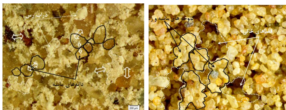
شکل ۱۵. تصویر میکروسکوپی ترکیب ماسه با ۱۰ درصد ریزدانه خمیری با روش WT (بزرگ‌نمایی ۱۶ برابر) شکل ۱۶. تصویر میکروسکوپی ترکیب ماسه با ۱۰ درصد ریزدانه خمیری با روش DD (بزرگ‌نمایی ۴۰ برابر)
