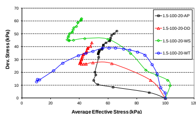
شکل ۹. نمودارهای مسیر تنش ترکیبیات ماسه و رس (1.5-100-20-WT;DD;WS;AP)
