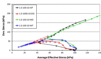
شکل ۷. نمودارهای مسیر تنش ترکیبیات ماسه و رس (1.5-100-10-WT;DD;WS;AP)
