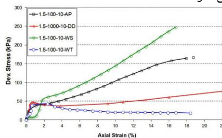
شکل ۶. نمودارهای تنش کرنش محوری ترکیبیات ماسه و رس (1.5-100-10-WT;DD;WS;AP)
