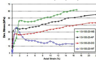
شکل ۸. نمودارهای تنش کرنش محوری ترکیبیات ماسه و رس (1.5-100-20-WT;DD;WS;AP)
