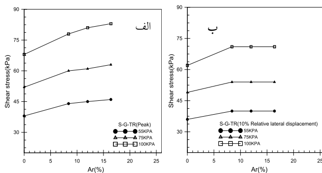
شکل ۱۷. تغییر تنش برشی در تنش‌های قائم مختلف برای آزمایش S-G-TR به‌ازای نسبت ناحیه اصلاح شده مختلف (الف) حالت حداکثر، (ب) حالت متناظر با جابه‌جایی افقی ۱۰ درصد
