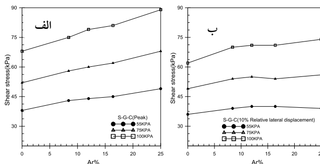
شکل ۱۵. تغییر تنش برشی در تنش‌های قائم مختلف برای آزمایش S-G-C به‌ازای نسبت ناحیه اصلاح شده مختلف (الف) حالت حداکثر، (ب) حالت متناظر با جابه‌جایی افقی ۱۰ درصد
