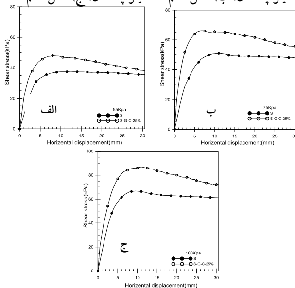
شکل ۱۴. نمودار جابه‌جایی افقی - تنش برشی در نسبت ناحیه اصلاح شده ۲۵ درصد الف) تنش قائم ۵۵ کیلو پاسکال، ب) تنش قائم ۷۵ کیلو پاسکال، ج) تنش قائم ۱۰۰ کیلو پاسکال
