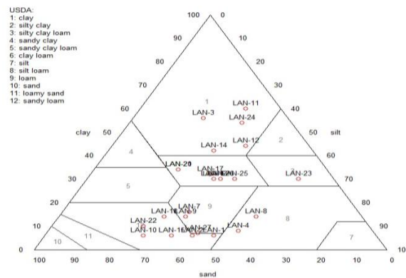
شکل ۳. نمودار مثلی بافت خاک‌های محل دفن زباله
