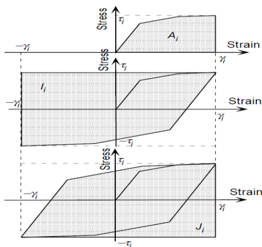
شکل ۶. مساحت‌های A_i ، I_i و J_i برای محاسبه حلقه هیستریک مدل IM در طول چرخه بارگذاری و باربرداری [۱۱]
