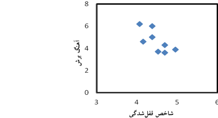
شکل ۱۱. ارتباط بین شاخص قفل‌شدگی و آهنگ برش
