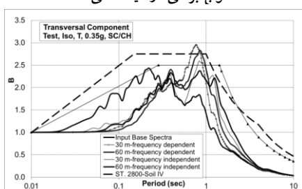
د) PGA=0.35g ، خاک نوع IV، مبنا سرعت
