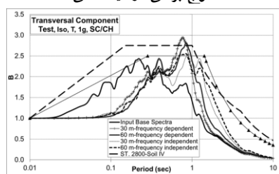
ی) PGA=1g ، خاک نوع IV، مبنا سرعت موج
