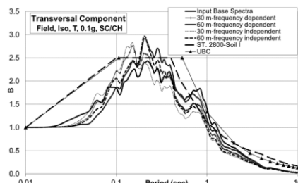
الف) PGA=0.1g ، خاک نوع I، مبنا سرعت موج
