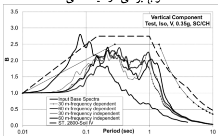
د) PGA=0.35g ، خاک نوع IV، مبنا سرعت موج برشی آزمایشگاهی
