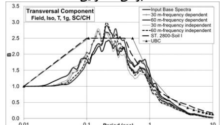
ه) PGA=1g ، خاک نوع I، مبنا سرعت موج برشی
