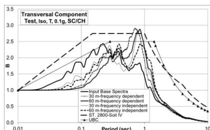
ب) PGA=0.1g ، خاک نوع IV، مبنا سرعت
