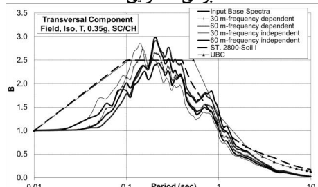
ج) PGA=0.35g ، خاک نوع I، مبنا سرعت موج
