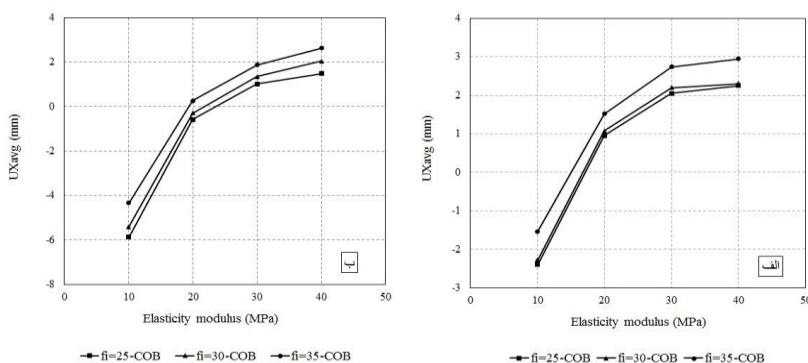
شکل ۸. مدول الاستیسیته- جابه‌جایی میانگین برای تراز آب الف) ۰، ب) ۲۵ متری از سطح زمین
