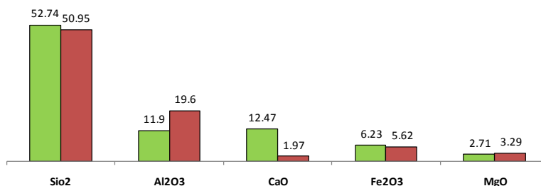
شکل ۱۱. مقایسه درصد اکسیدهای نانورس استفاده شده با میانگین ترکیب لس‌های استان
