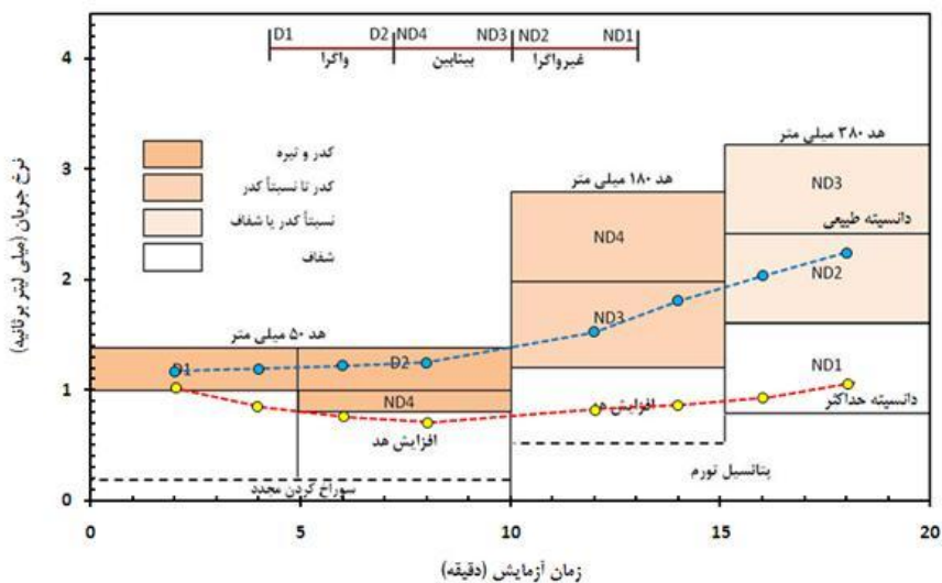
شکل ۹. نتایج نرخ جریان در زمان‌های مختلف آزمایش روی خاک منطقه بقچه‌بالا
