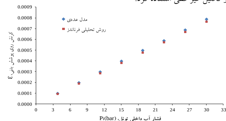
شکل ۴. مقایسه نتایج تحلیل کرنش روی پوشش بتنی
