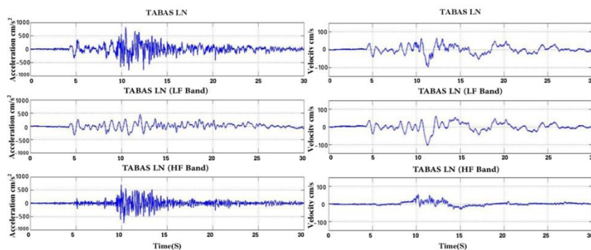
شکل ۳. تاریخچه زمانی شتاب و سرعت متناظر با مؤلفه LN از رکورد اصلی زلزله TABAS، نمایش تاریخچه زمانی سرعت متناظر با بخش‌های فرکانس پایین (LF) و فرکانس بالا (HF)، نمایش تاریخچه زمانی سرعت متناظر با بخش فرکانس پایین شباهت زیادی با تاریخچه اصلی دارد.
