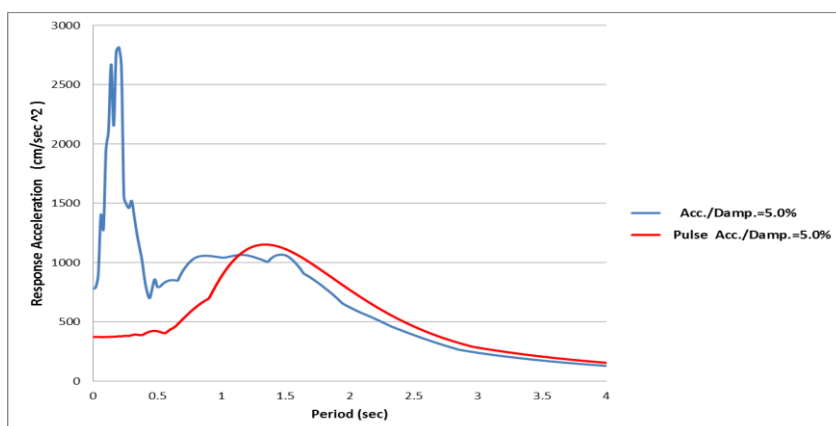
شکل ۱۰. مقایسه طیف پاسخ شتاب مؤلفه TR رکورد اصلی و مدل پایه ریاضی BAM 2003
