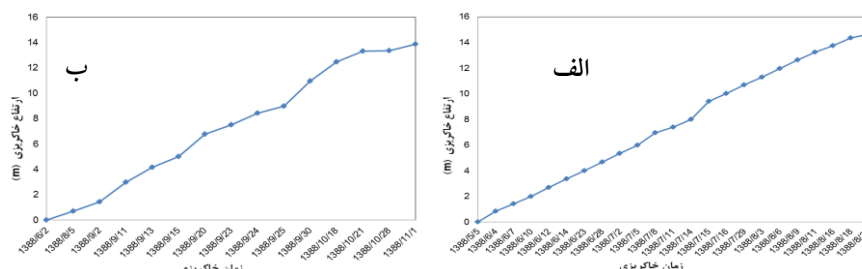
شکل ۱۱. الف) نمودار تاریخچه خاکریزی خاکریز EM-2B، ب) نمودار تاریخچه خاکریزی EM-3
