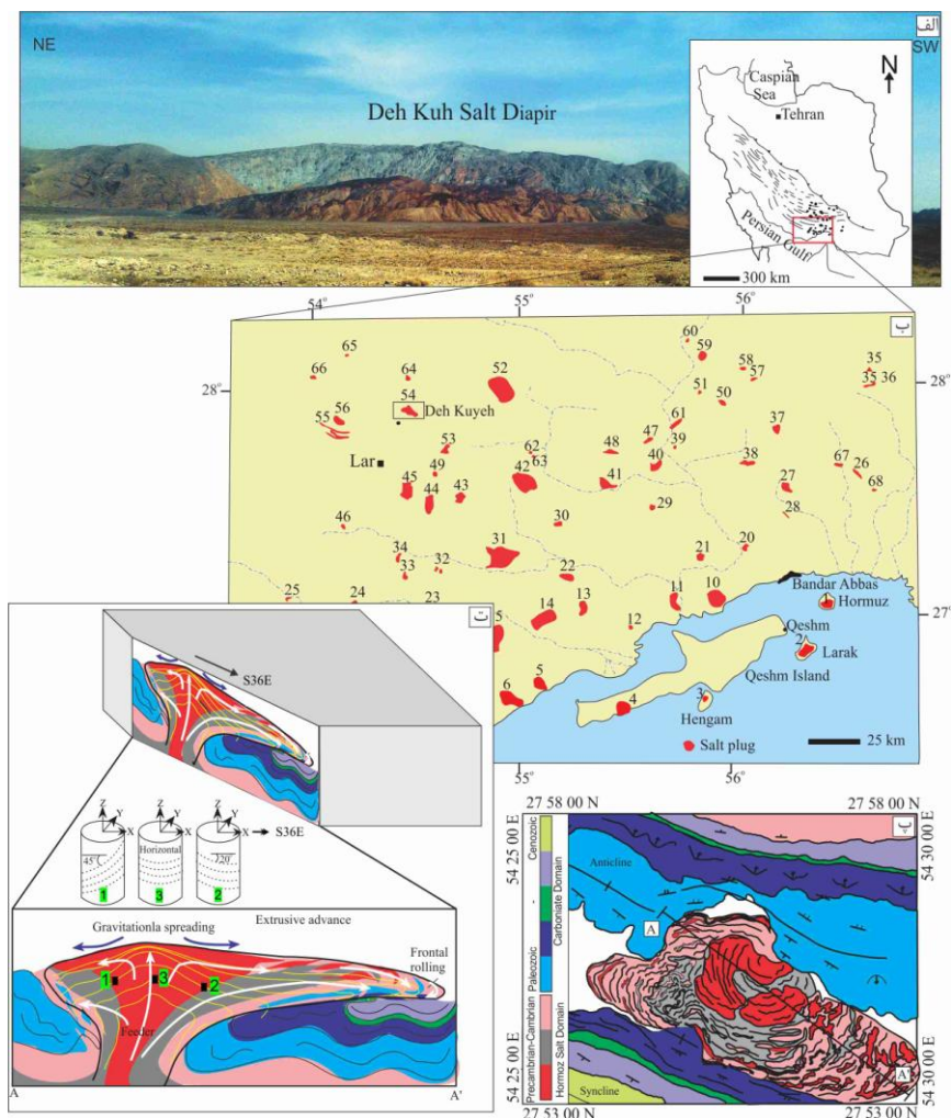
شکل ۱. الف) نمای از دیاپیر نمکی دهکویه، ب) موقعیت دیاپیرهای نمکی شناسایی شده در زاگرس و خلیج فارس، پ) نقشه زمین شناسی دیاپیر نمکی دهکویه، ت) برش ختاری از موقعیت AA' در نقشه زمین شناسی (تصویر پ)
