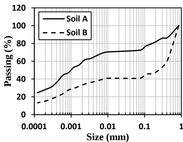
شکل ۳. منحنی دانه‌بندی خاک‌های واگرای استفاده شده در این تحقیق
