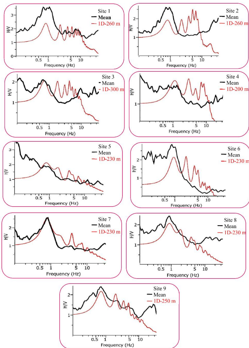
شکل ۹. مقایسه نتایج بزرگ‌نمایی حاصل از میکروترمورها و مدل‌سازی یک‌بعدی با در نظر گرفتن سنگ بستر با سرعت ۱۳۰۰ متر بر ثانیه در عمق ۲۰۰ تا ۳۰۰ متر
