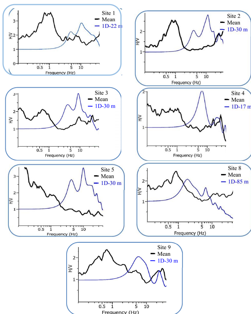
شکل ۶. مقایسه توابع بزرگ‌نمایی حاصل از میکروترموورها و مدل‌سازی یک‌بعدی با در نظر گرفتن سنگ بستر با سرعت ۷۶۰ متر بر ثانیه و عمق کم آبرفت (۱۷ تا ۳۰ متر)
