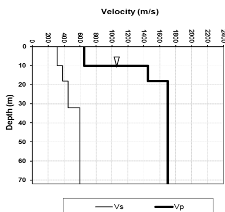
شکل ۵. تغییرات سرعت موج فشاری و برشی در گمانه A09 ساختگاه ۸ با آزمایش‌های درون چاهی
