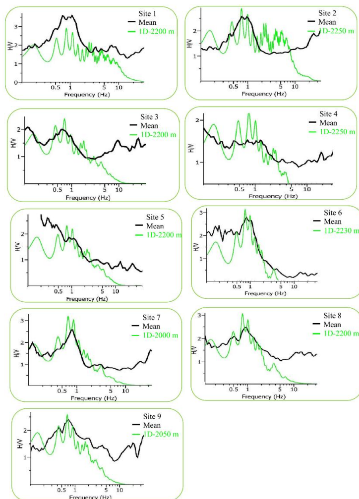
شکل ۱۰. مقایسه توابع بزرگ‌نمایی حاصل از میکروترموورها و مدل‌سازی یک‌بعدی با در نظر گرفتن پی سنگ با سرعت ۲۵۰۰ متر بر ثانیه در عمق ۲۰۲۰ تا ۲۲۵۰ متر
