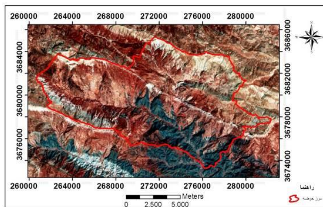
شکل ۲. ترکیب باندی ۵۳۲ حوضه وارک
