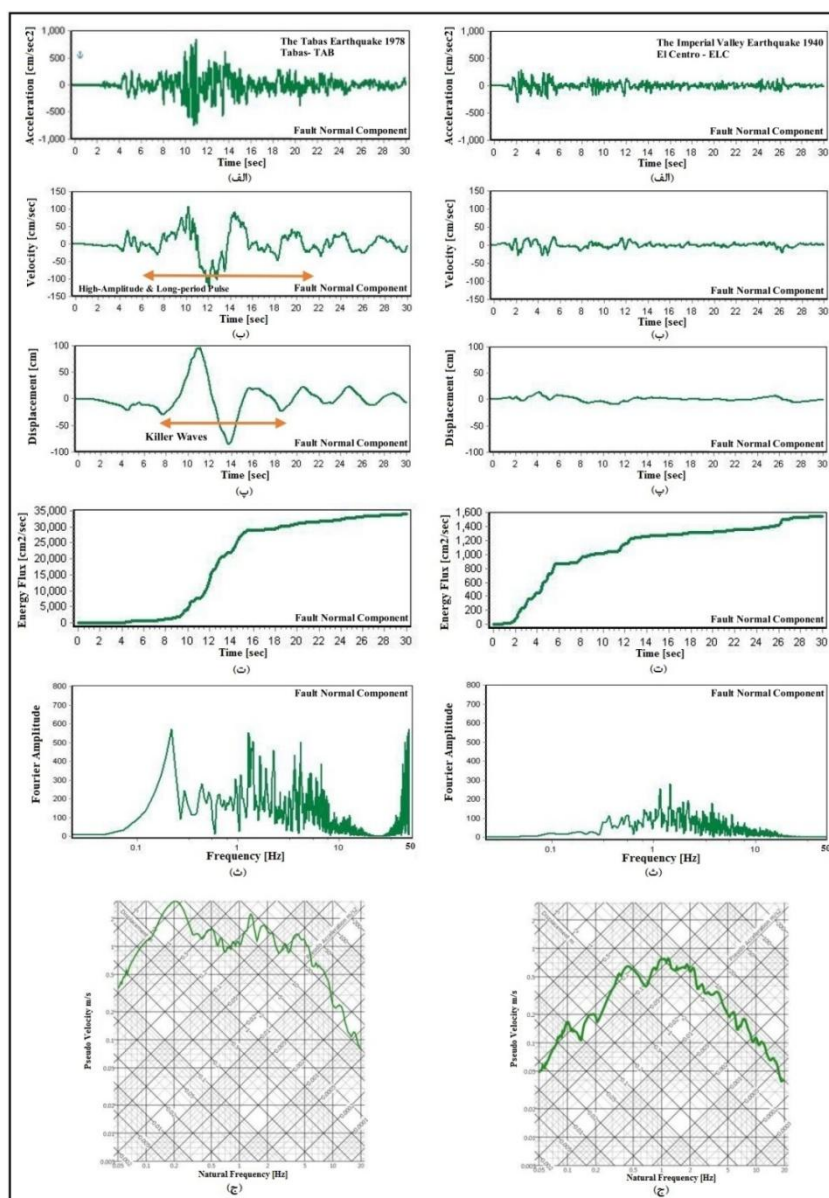
شکل ۱. مشخصات رکورد حوزه دور ELC شکل ۲. مشخصات رکورد حوزه نزدیک TAB متناظر با مولفه عمود بر صفحه شکست متناظر با مولفه عمود بر صفحه شکست گسل از زلزله کالیفرنیا El Centro 1940 گسل از زلزله Tabas 1978
