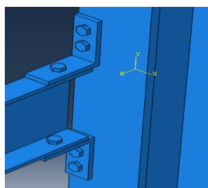
شکل ۴. اتصال نبشی نشیمن ساده پیچی (e)
