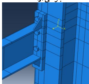
شکل ۱۰. اتصال با ورق انتهایی و لچکی (l)
