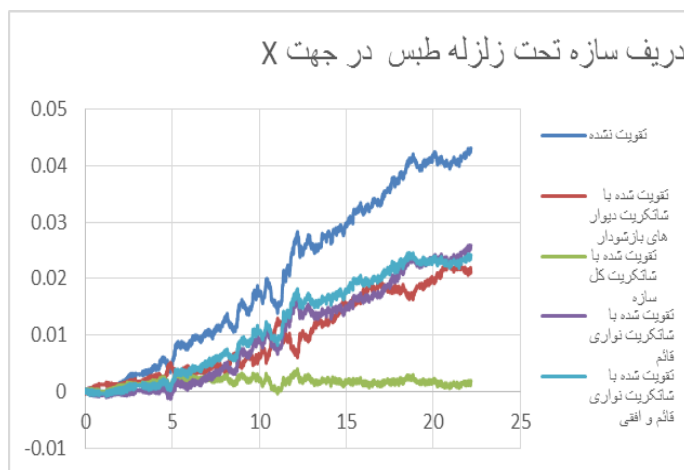
شکل ۱۲. ب) نمودار دررفت سازه تحت زلزله طبس در جهت X
