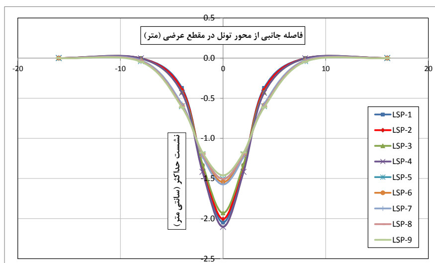
شکل ۶. منحنی‌های گودی نشست (پیش‌بینی شده) در مقاطع عرضی برای نقاط بررسی شده [۱]
