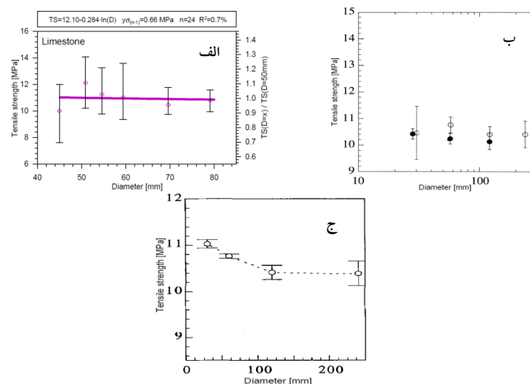
شکل ۱. پژوهش‌های انجام شده در زمینه تأثیر قطر نمونه بر مقاومت کششی برزیلی؛ الف) پژوهش‌های گویینی و همکاران [۳۹] روی نمونه‌های گرانیتی، ب) پژوهش‌های روکو و همکاران [۱۴] روی نمونه‌های گرانیتی، ج) پژوهش‌های تورو و همکاران [۴۲] روی نمونه‌های سنگ آهک
