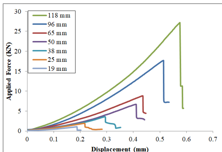
شکل ۷. منحنی نیرو- جابه‌جایی برای نمونه‌ها با قطرهای مختلف
