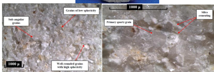
شکل ۳. الف) مقطعی از نمونه تهیه شده به قطر ۵۰ میلی‌متر، ب) نمایش توزیع و شکل دانه‌های اولیه کوارتز با مقیاس ۱۰۰۰ میکرون و ج) سیمان‌شدگی سیلیکاته دانه‌های اولیه با مقیاس ۱۰۰۰ میکرون
