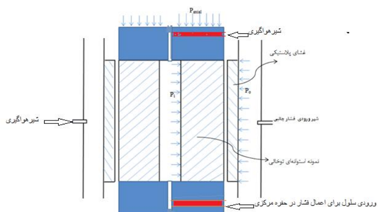
شکل ۳. نمایی از طراحی انجام شده برای اعمال فشار داخلی در سلول هوک تغییر یافته (در شکل نشان‌دهنده تنش محوری، P_{axial} نشان‌دهنده تنش جانبی و P_o نشان‌دهنده فشار در حفره مرکزی است)
