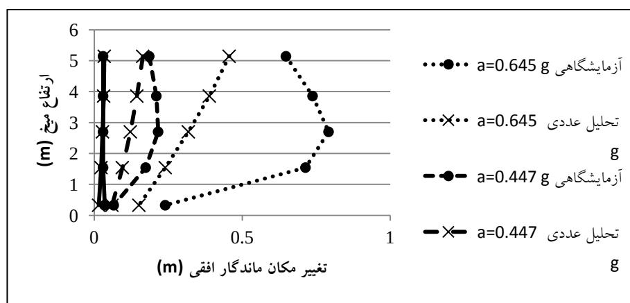
شکل ۴. نتایج تحلیل عددی و آزمایشگاهی میز لرزان
