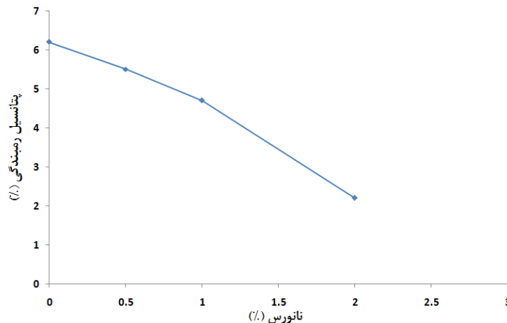
شکل ۱۲. تأثیر افزودن نانورس بر پتانسیل رېمېندگي نمونه‌های خاک اینچه‌برون
