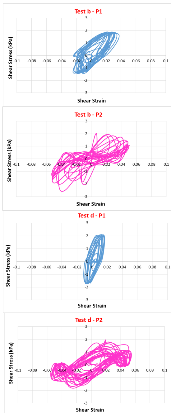
شکل ۷. رفتار تنش-کرنش برشی در عمق درموقعیت‌های P1 و P2 برای تست‌های TC_r = 10\% (b) و TC_r = 20\% (d)
