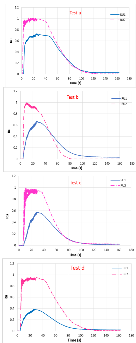
شکل ۵. نسبت اضافه فشار آب حفره‌ای ( R_u ) برای تست‌های مدل
