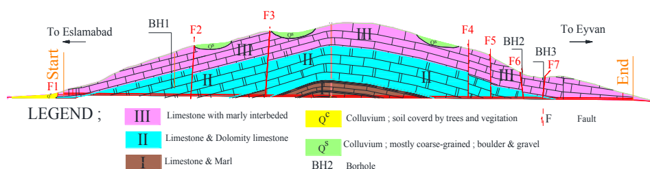
شکل ۲. پروفیل طولی زمین‌شناسی تونل قلاجیه
