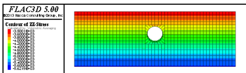
شکل ۶. کانتور تنش‌های قائم، قبل از شروع برخواست لوله
