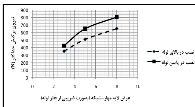
شکل ۱۶. نحوه تغییرات مقاومت برخواست لوله با عرض لایه مهر-شبكة به صورت نصب در بالا و پایین لوله
