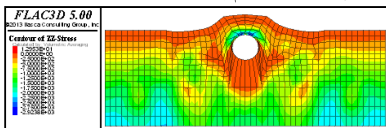
شکل ۸. کانتور تنش‌های قائم، پس از اعمال ۲۰۰ نیوتن نیروی برخواست لوله
