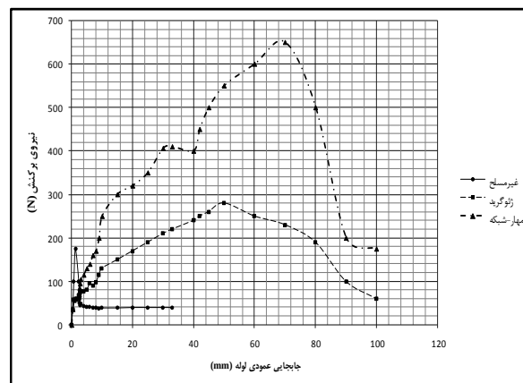
شکل ۱۱. تغییرات نیروی برخاست حداکثر در برابر جابجایی عمودی لوله در ماسه خشک ( D=50\text{ mm} , N=1 , h/D=2 , b=5D )
