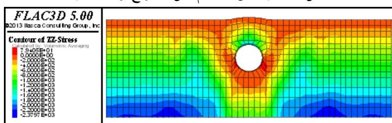
شکل ۷. کانتور تنش‌های قائم، پس از اعمال ۱۴۰ نیوتن نیروی برخواست لوله
