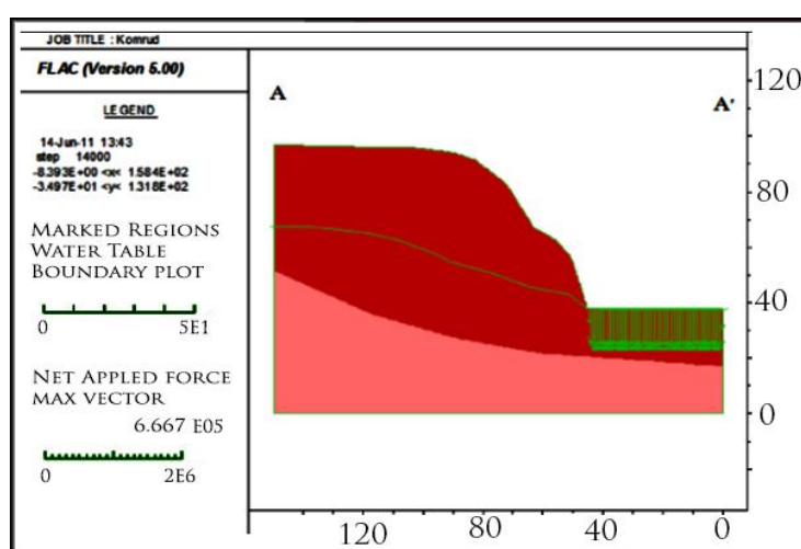
شکل ۱۵. مقطع تیپ هندسه شیروانی کمرود، سنگ کف به رنگ صورتی، مصالح خاکی قرمز رنگ، سطح فراطیک با خط سبز و تنش وارد بر پاشنه شیروانی با پیکان سبز نشان داده شده است. جدول ۴. خصوصیات خاک مقطع تیپ.
