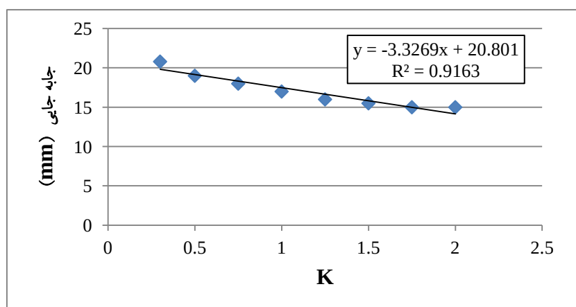
شکل ۸. نمودار تأثیر تغییرات تدریجی K بر جاب‌جایی عمودی سقف
