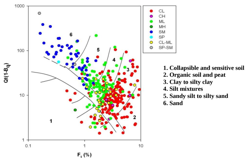
شکل ۹. طبقه‌بندی خاک با استفاده از روش جفری و دویس [۱۲] و مقایسه آن با نتایج آزمایش دانه‌بندی در تحقیق حاضر
