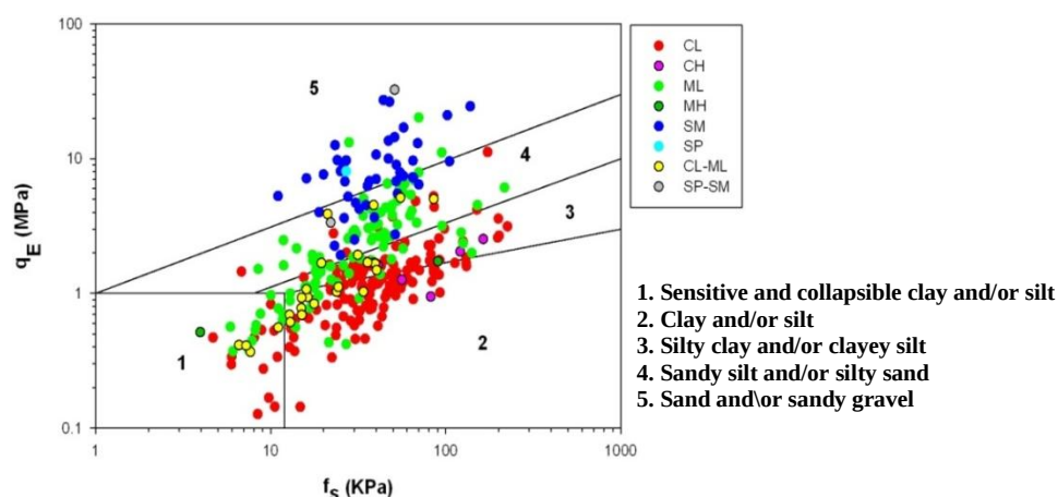
شکل ۱۰. طبقه‌بندی خاک با استفاده از روش اسلامی و فلیوس [۱۳] و مقایسه آن با نتایج آزمایش دانه‌بندی در تحقیق حاضر
