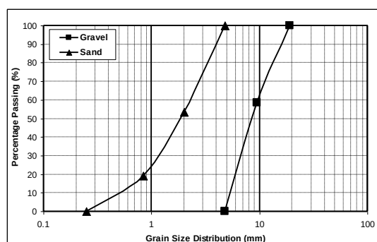
شکل ۴. دانه‌بندی مصالح داسیت بررسی شده
