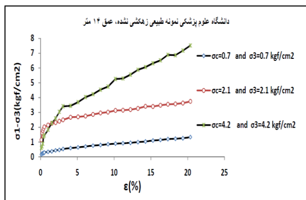
شکل ۲۲. منحنی‌های تنش- کرنش محوری نمونه‌های طبیعی زهکشی نشده، دانشگاه علوم پزشکی نمونه طبیعی زهکشی نشده، عمق ۱۴ متر
