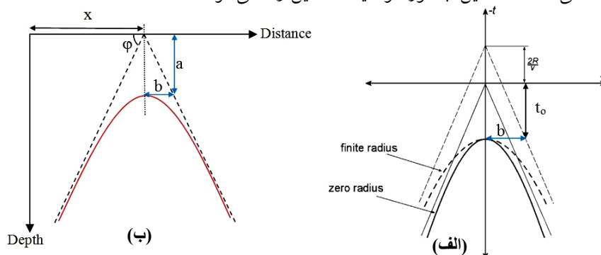
شکل ۳. الف) تعریف پارامترهای مشخصه هذلولی در حوزه مکان- زمان، ب) پاسخ تپیک GPR به صورت هذلولی برای هدف، همراه با نمایش پارامترهای هندسی آن در حوزه مکانی
