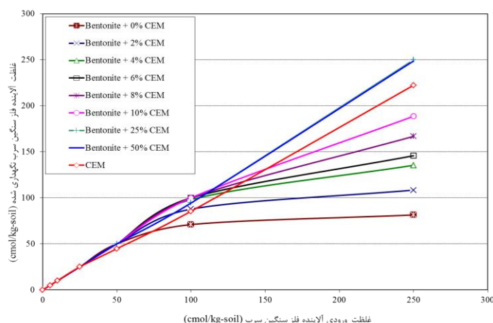
شکل ۳. قابلیت نگهداری آلایندۀ فلز سنگین سرب با نمونه رسی بتونیت اصلاح شده با درصد‌های مختلف سیمان
