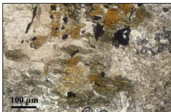
شکل ۴. عکس میکروسکوپی مقطع نازک سنگ با نور طبیعی (فتو کریست‌های آمفیبول در زمینه‌ای از شیشه)
