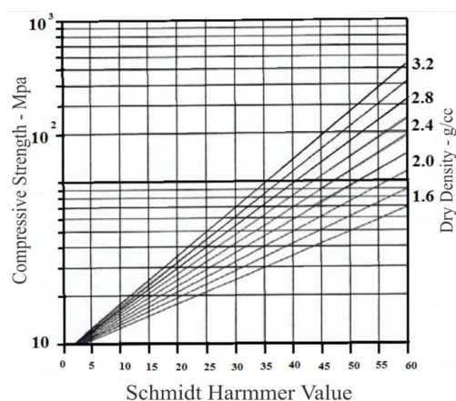
شکل ۱۲. رابطه بین مقدر عددی چکش اشمیت و مقاومت فشاری تک‌محوره به‌عنوان تابعی از چگالی خشک (دیر و میلر، ۱۹۶۵ نقل از فهیمی‌فر و سروش، ۱۳۸۰)
