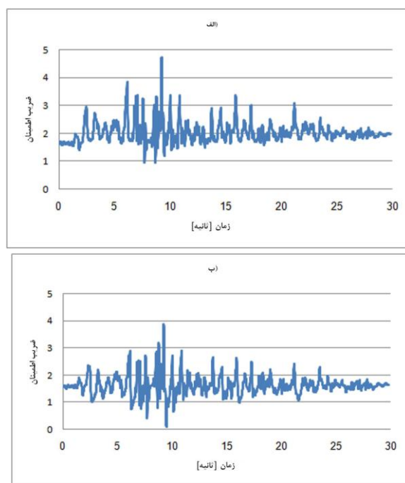
شکل ۱۰. تاریخچه زمانی ضریب اطمینان معادل تغییر مکان مجاز گوه در زلزله طبس مقیاس شده به 0.64g (الف) قبل از اعمال فیلتر بالاگذر (ب) پس از اعمال فیلتر بالاگذر
