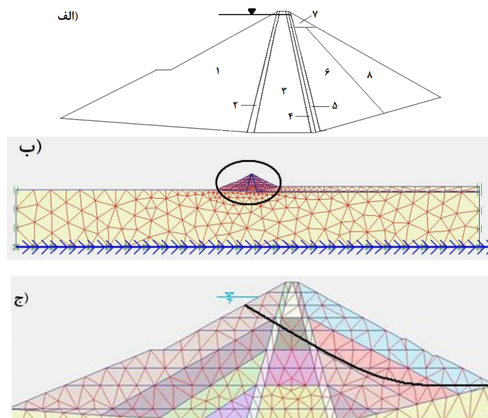
شکل ۲. الف) مقطع سد مسجدسلیمان به همراه نواحی مختلف مصالح ب) شبکه اجزا محدود بدنه و فونداسیون سد مسجدسلیمان ج) قسمت بزرگ شده بدنه سد و بحرانی‌ترین گوه مستعد لغزش
