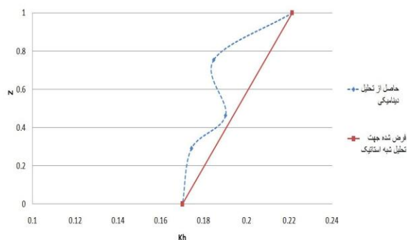
شکل ۱۳. ضریب شتاب افقی متغیر در ارتفاع سد مسجدسلیمان
