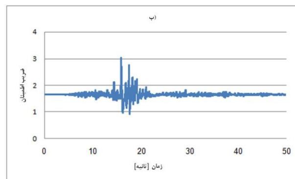
شکل ۶. تاریخچه زمانی ضریب اطمینان گوه مستعد لغزش در حالت تحریک با زلزله چپ چپ (الف) قبل از اعمال فیلتر بالاگذر (ب) پس از اعمال فیلتر بالا گذر
