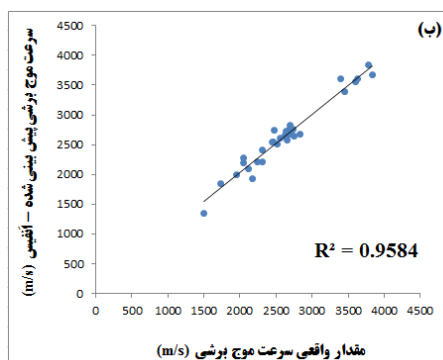
شکل ۵. ضریب تعیین ( R^2 ) بین مقادیر واقعی سرعت موج برشی و پیش‌بینی‌های آنفیس (الف: فاز آموزش؛ ب: فاز آزمایش)
