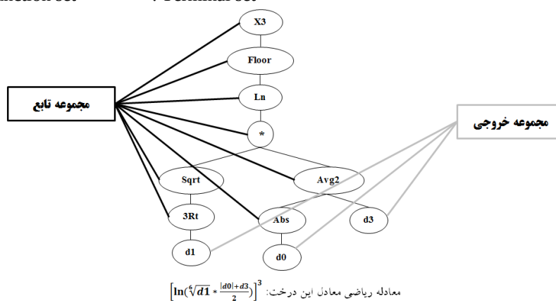
شکل ۳. نمونه‌ای از نمودار درختی به‌دست آمده در جپ و تابع ریاضی مربوط به آن [۲۳]
