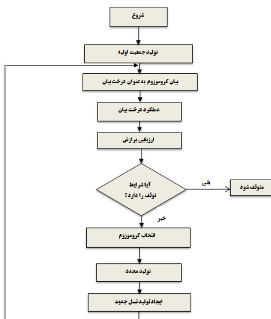
شکل ۲. الگوریتم جپ [۲۵]
