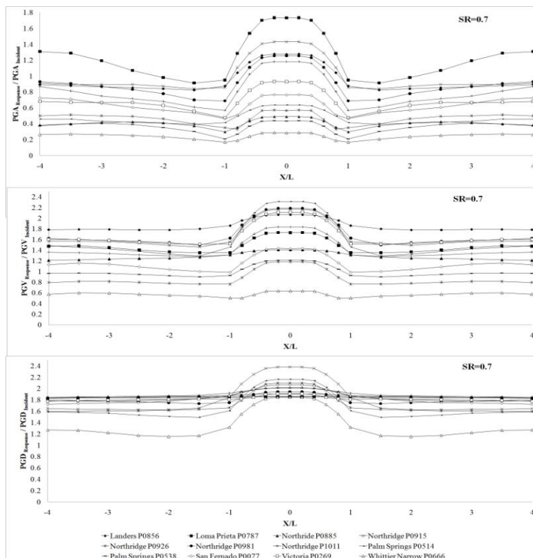
شکل ۸. نمودارهای بزرگنمایی مؤلفه‌های افقی شتاب، سرعت و جابه‌جایی در فاصله‌های بی‌بعد شده از مرکز تپه به‌ازای ۱۲ رکورد زلزله برای تپه‌ای با ضریب شکل ۰/۷ و نسبت میرایی ۰/۵. این بار نتایج تحلیل میدان آزاد، مقادیر بزرگنمایی کم‌تری نسبت به تحلیل دوبعدی به‌دست می‌دهند. از این رو، استفاده از نتایج تحلیل دوبعدی در این ناحیه ضرورت پیدا می‌کند.
