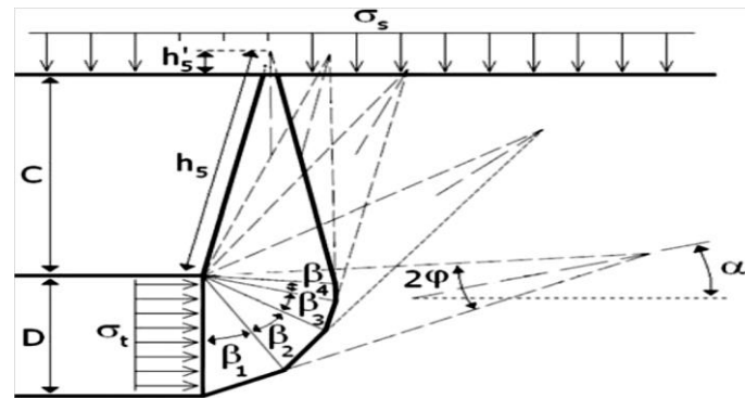
در سال ۲۰۱۰ سوبارا و همکاران، روش لکا و دورمیو (۱۹۹۰) و مولن و همکاران (۲۰۰۹) را بهبود بخشیدند. در واقع آن‌ها مکانیسمی را پیشنهاد دادند که در آن تمام جبهه تونل (دایره کامل) ریزش می‌کند، بر خلاف مکانیسم‌های قبلی که فقط یک مقطع بیضوی از کل جبهه ریزش می‌کند. مولن (۲۰۰۹) در نتایجی که به‌دست آورد نشان داد که برای یک مکانیسم پنج بلوکی ( n=5 )، شواهد کافی وجود دارد که افزایش تعداد بلوک‌ها به بیش از ۵ عدد، تنها باعث ۱٪ بهبود در دقت جواب‌ها می‌گردد [۱۵]. هم‌چنین سوبارا و همکاران (۲۰۱۰) با بررسی‌هایی که بر روی سه نمونه خاک مختلف انجام دادند به این نتیجه رسیدند که مکانیسم تک بلوکی تنها برای خاک بدون چسبندگی ( c=0 ) و برای مقادیر بزرگی از زاویه اصطکاک داخلی ( \phi = 40^\circ ) به‌کار برود چرا که افزایش تعداد بلوک‌های مخروطی در این نوع از خاک‌ها مقدار فشار اعمالی بر جبهه تونل را به‌صورت بسیار ناچیزی بهبود می‌بخشد (کم‌تر از ۱ درصد)، از این رو مکانیسم شکست مذکور استفاده شد. این محققان با بررسی‌هایی که انجام دادند این پیشنهاد را دادند که برای به‌دست آوردن مقادیر N_C ، N_S و N_\gamma علاوه بر فرمول‌های مربوطه می‌توان از جدول ۱ نیز استفاده کرد که برای مقادیر مختلفی از \frac{c}{D} و \phi به‌دست آمده است.
