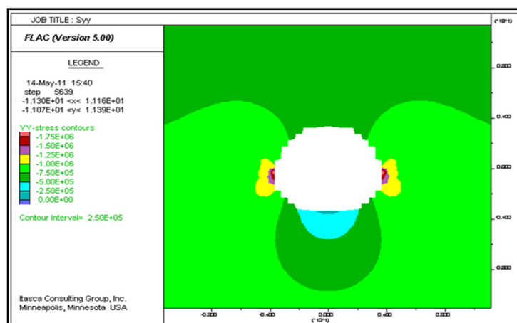
شکل ۱۰. کتور تنش Syy در اطراف تونل بعد از نصب سیستم نگه‌داری بنچینگ (مقطع ۳۰+۹۰۰)
