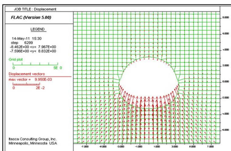
شکل ۹. بردارهای جابه‌جایی در اطراف تونل بعد از نصب سیستم نگهداری بنچینگ (مقطع ۳۰+۱۵۰)
