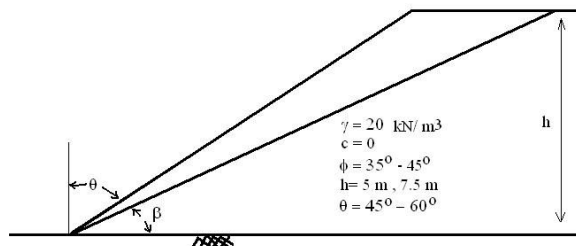
شکل ۵. شیب نمونه استفاده شده در تحلیل‌های لرزه‌ای
